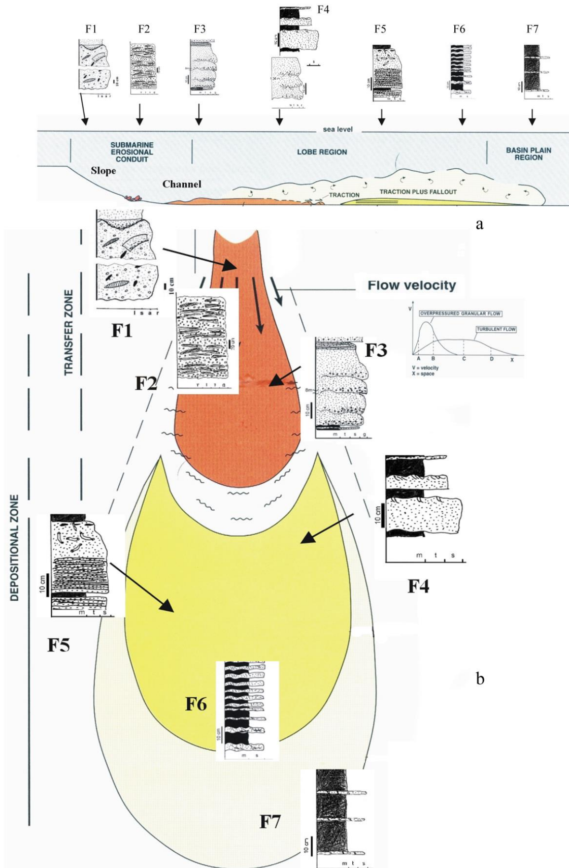
Fig. 9. Distribuția faciesurilor sedimentare: a – între taluz și câmpia bazinală; b – în cadrul zonelor de transfer depozitionale ale sistemului turbiditic în accepțiunea lui Mutti (1992).
