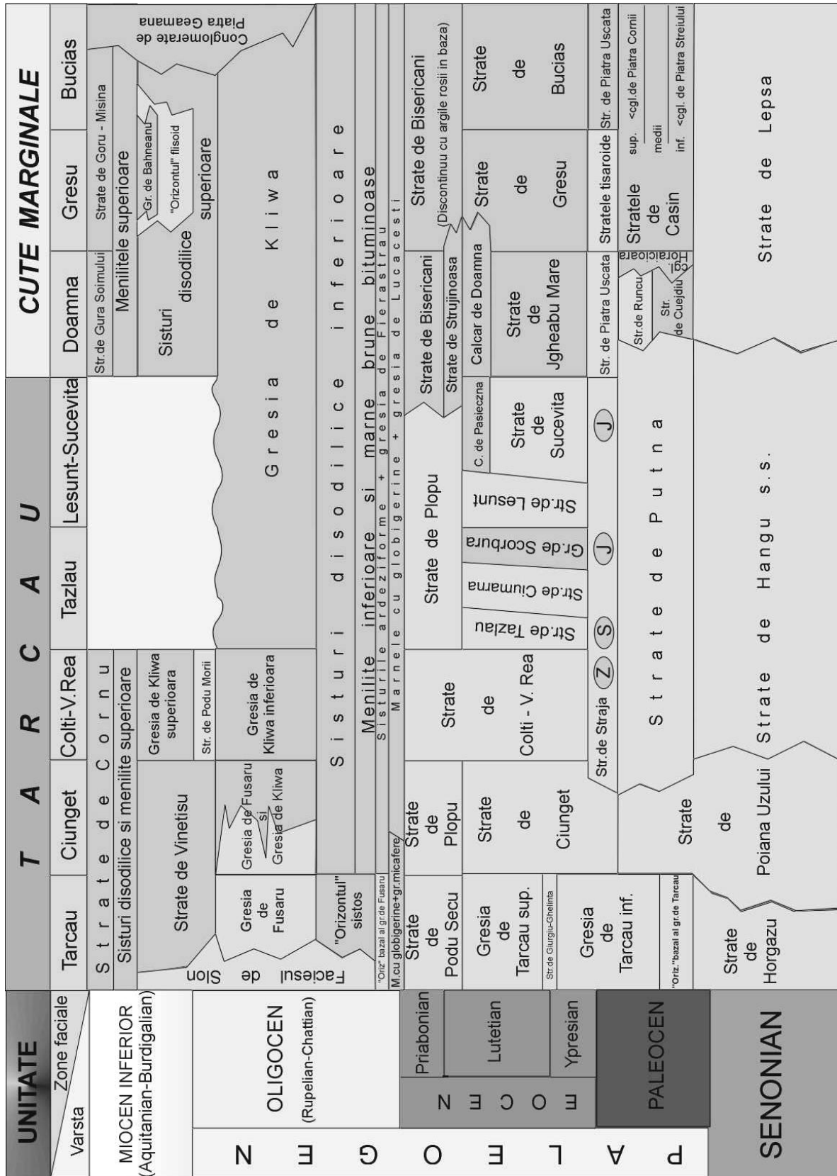
Fig. 2. Paralelizarea formațiunilor geologice din Moldavidele Carpaților Orientali.
