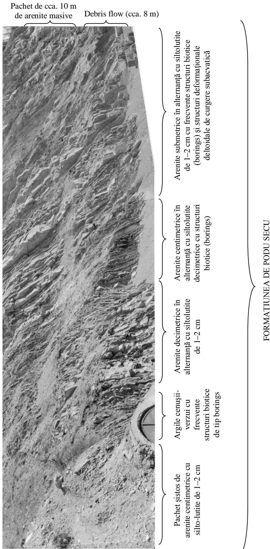
Fig. 5. Continuare fig.4 – imagine panoramică la topul Eocenului care surprinde contactul dintre Formațiunea gresiei de Tarcău și Formațiunea de Podu Secu – versantul stâng al văii Buzăului, aval de barajul Siriu, în curba drumului limitrof bazet deversorului barajului.
