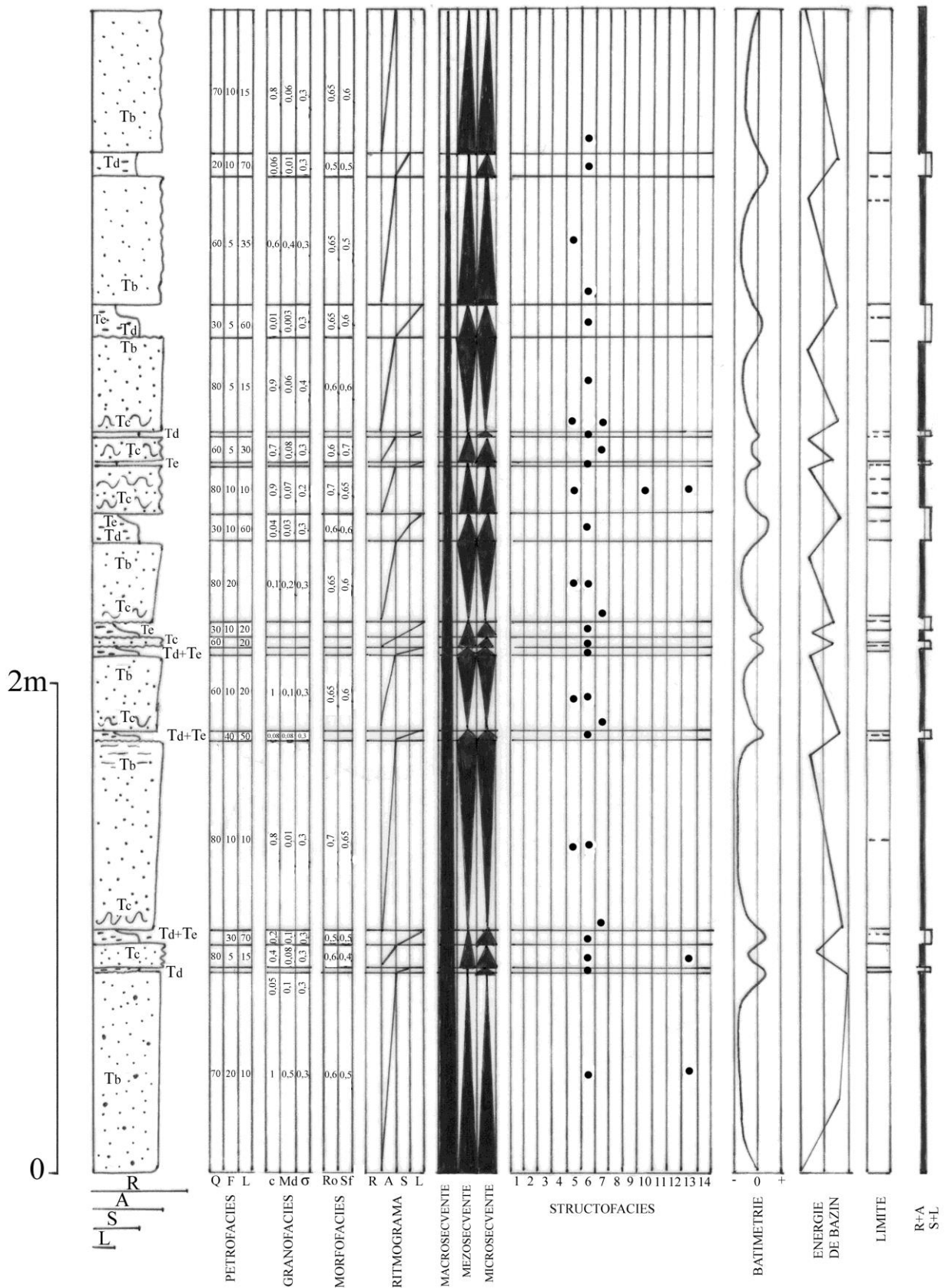
Fig. 8. Coloana sedimentologică a pachetului grezos, la cca. 10 m de la intrarea în galeria de vizitare de la baza barajului, în curba drumului limitrof deversorului de ape mari.
