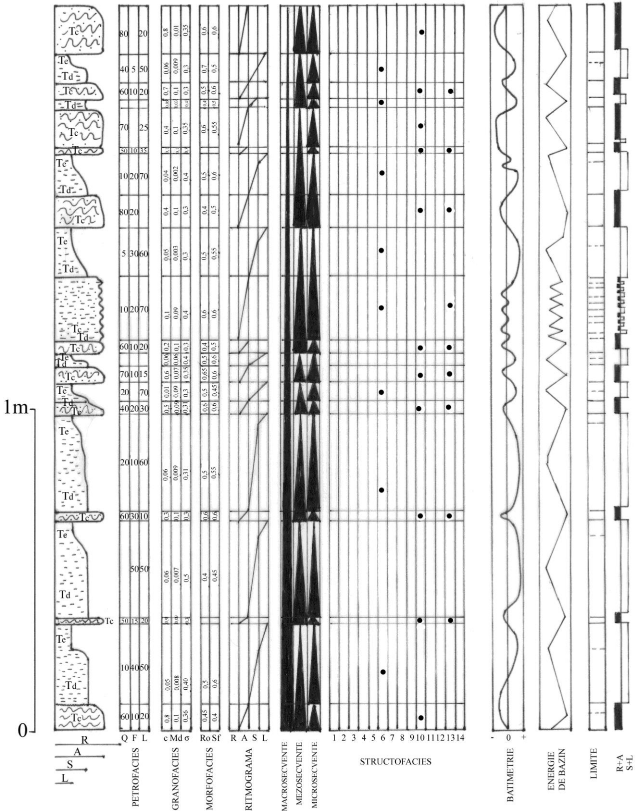
Fig. 7. Coloana sedimentologică a pachetului șistos-argilos cu intercalații grezoase, la cca. 4 m de la intrarea în galeria de vizitare de la baza barajului, în curba drumului limitrof deversorului de ape mari.
